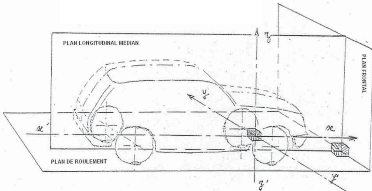
- Figure 3. Plans de référence -
