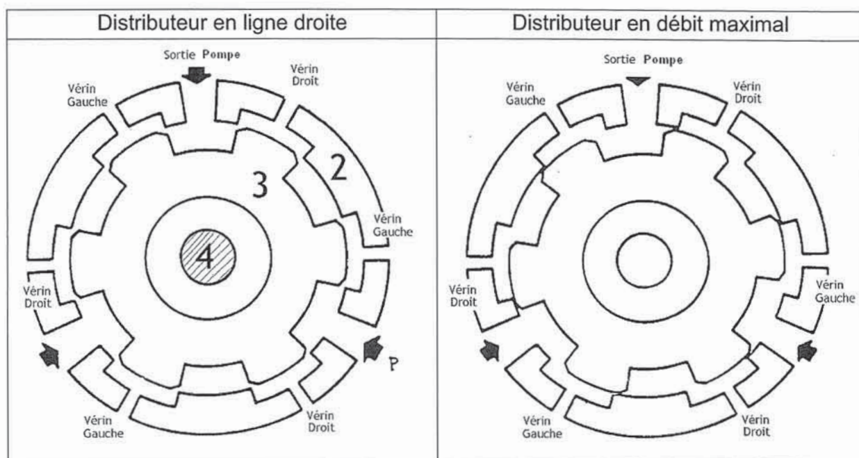
- Figure 11. Principe de fonctionnement de la valve -
