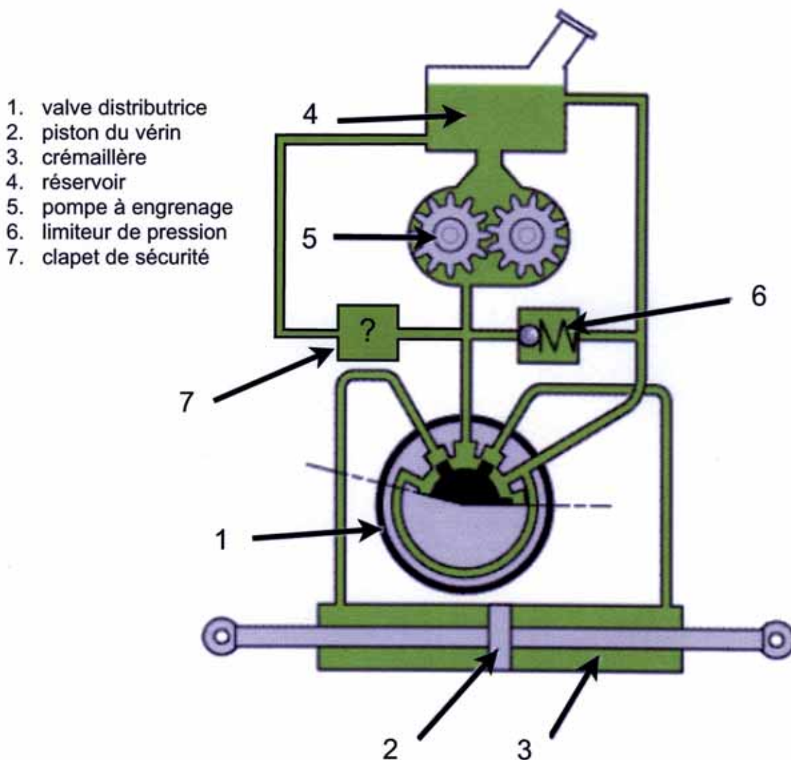
- Figure 5. Schéma hydraulique du système -
