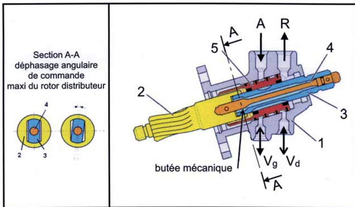
- Figure 10. Croquis technologique de la valve -
