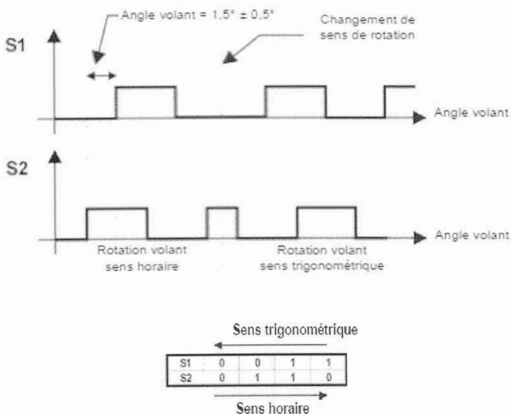
- Figure 15. Signaux délivrés par le capteur volant -
