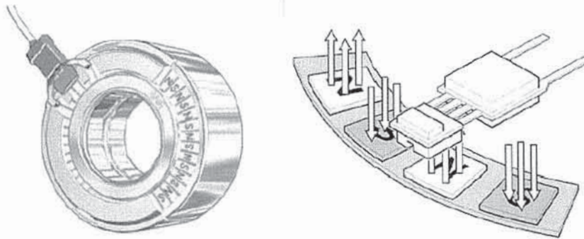
- Figure 14. Technologie du capteur de roue -
