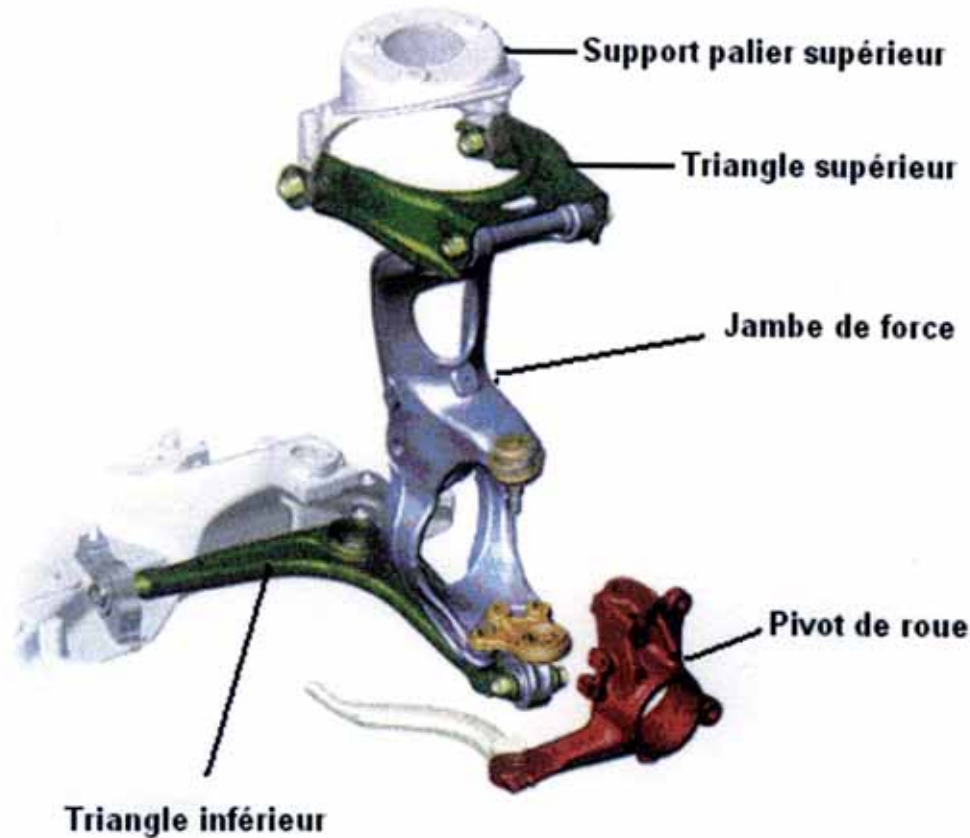
- Figure 2. Vue du train avant -
