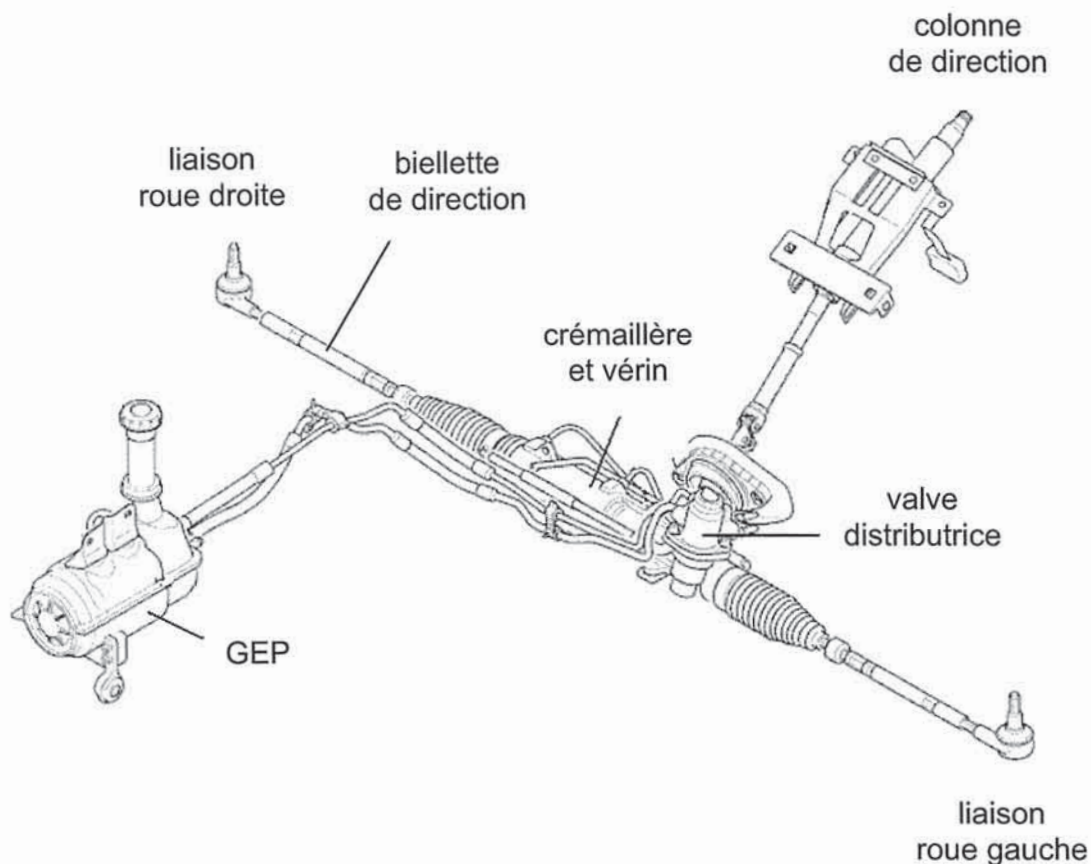
- Figure 1. Vue d'ensemble du système -
